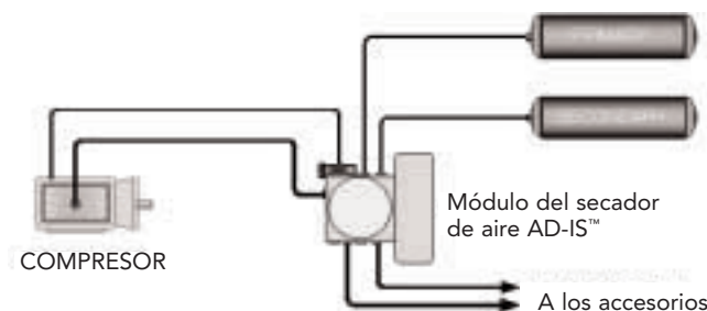
Esquema del secador de aire Bendix® AD-IS™
