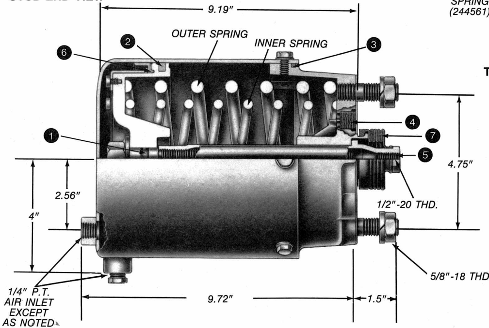
STUD END VIEW
